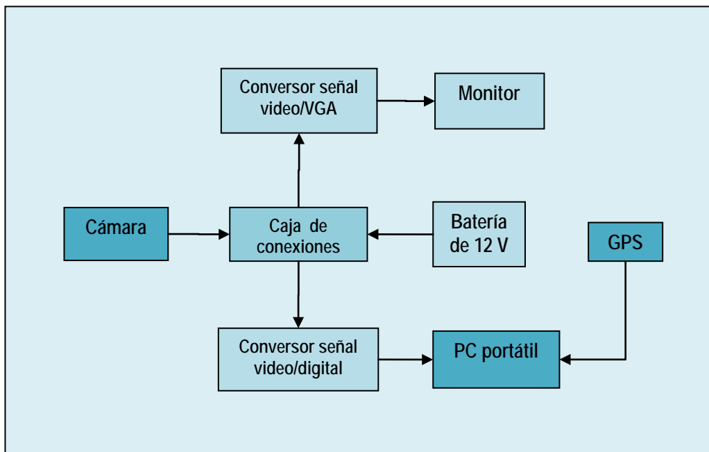
Figura 6. Esquema del sistema de circuito cerrado de televisión
