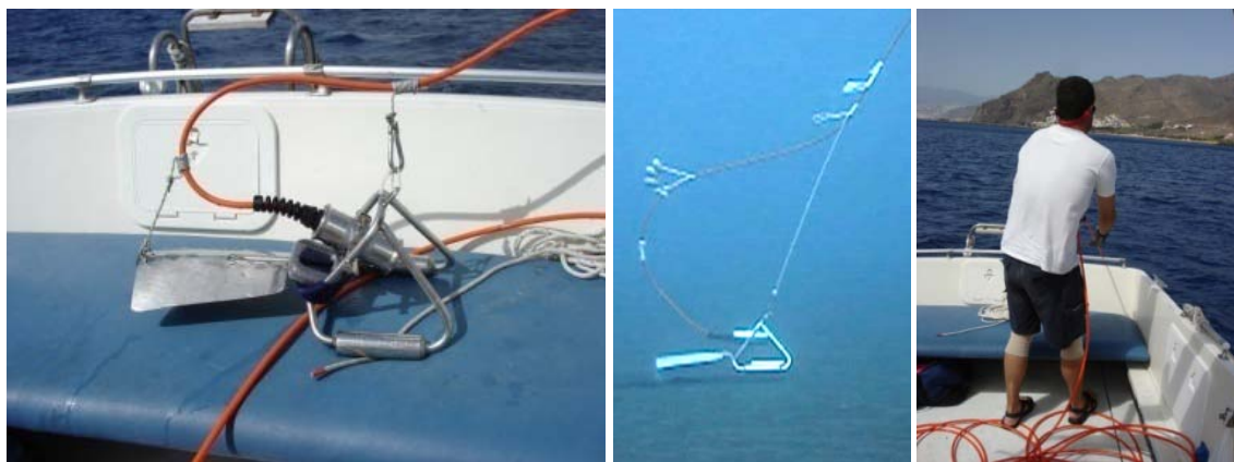
Figura 5. Izquierda: cámara de vídeo montada sobre patín.- Centro: deslizamiento del patín por el fondo marino. Derecha: sistema de arrastre controlado a mano para evitar colisiones.
