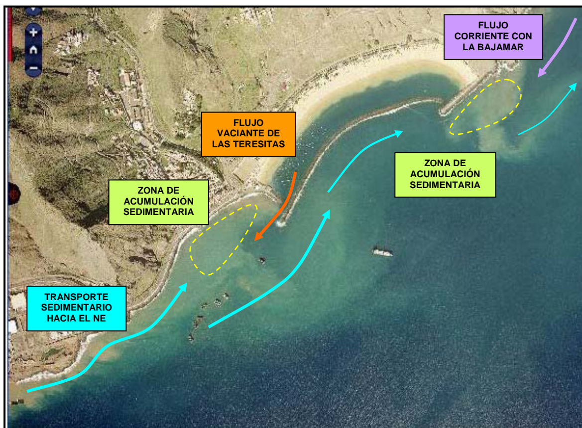
Figura 12. Observaciones sobre las corrientes y transporte sedimentario basado en una ortofoto de enero de 2002.
